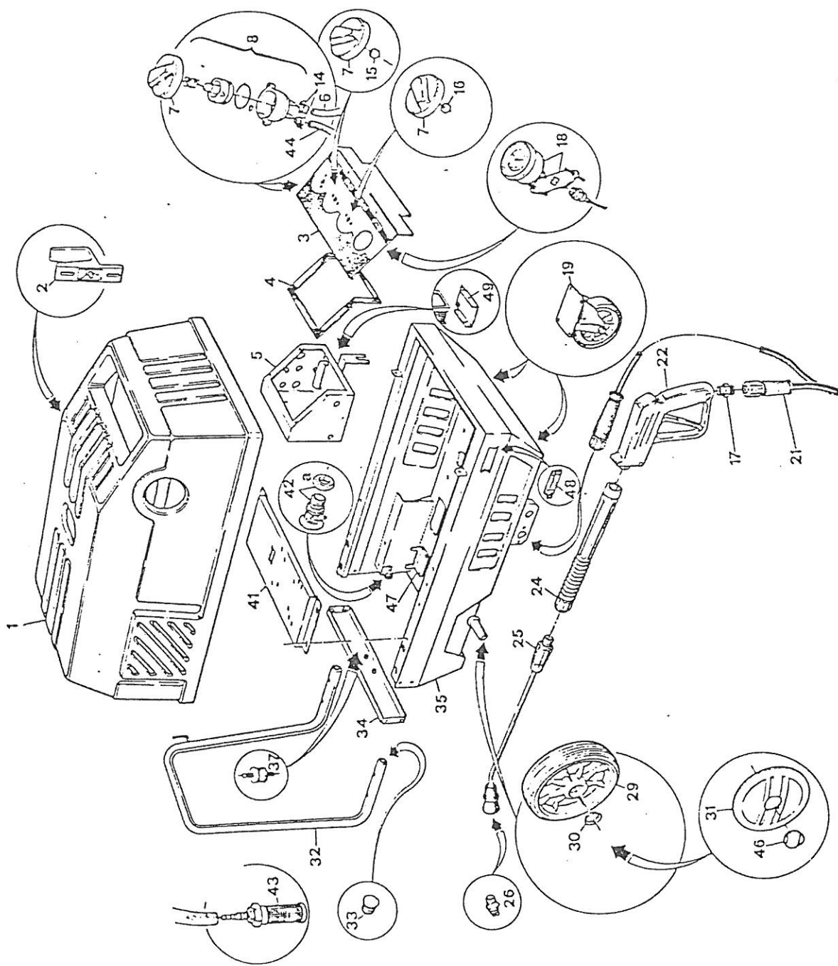
ERSATZTEILLISTE SUPER-JET HW 8100 IP
